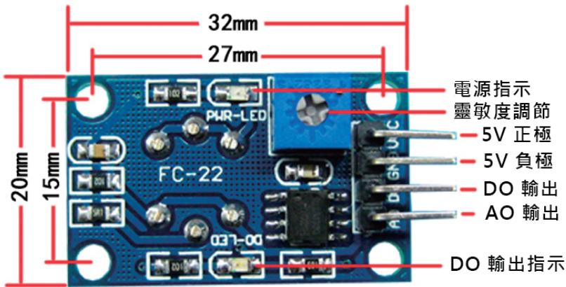
產品接線圖
